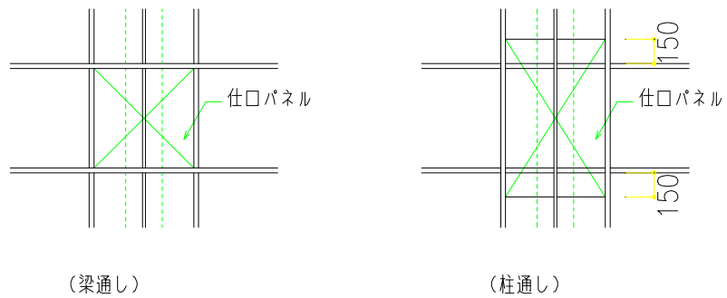
図4.1 仕口パネル
