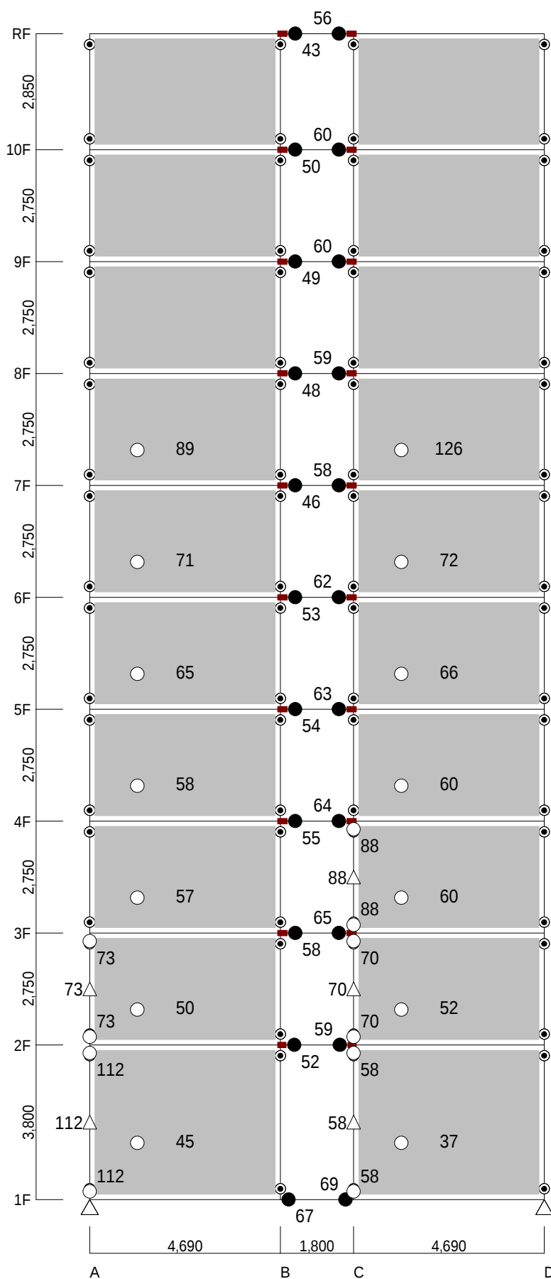
塑性ヒンジ発生図 :Y-方向 <5> フレーム :Y-方向左加力
