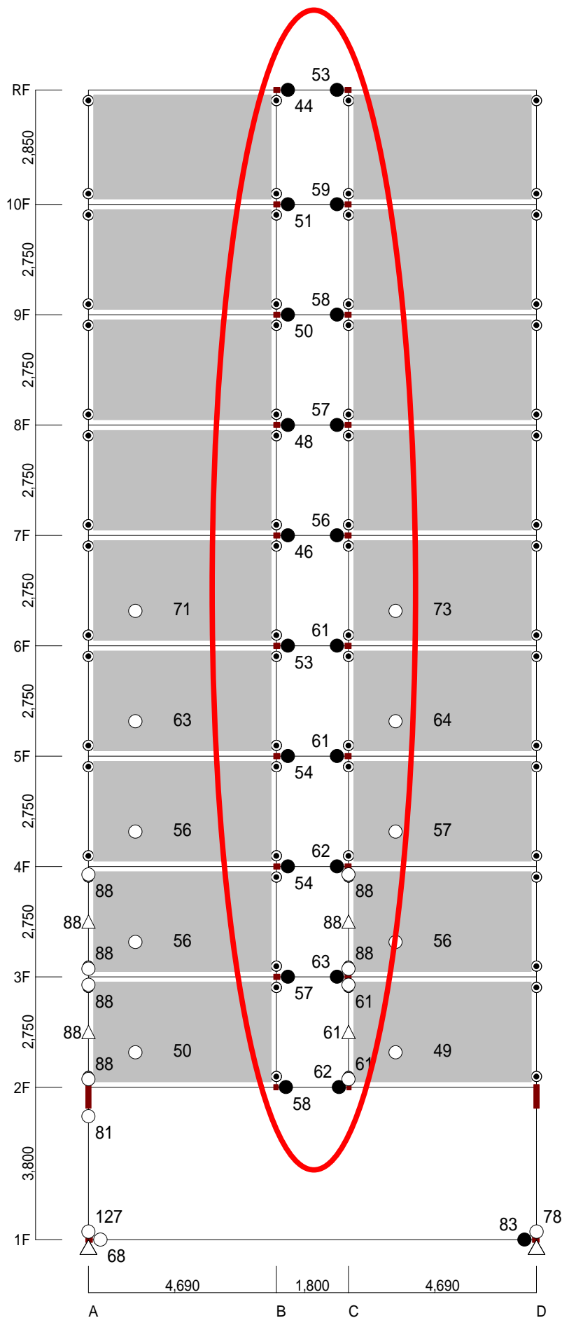
塑性ヒンジ発生図 :Y-方向 <2> フレーム :Y-方向左加力
