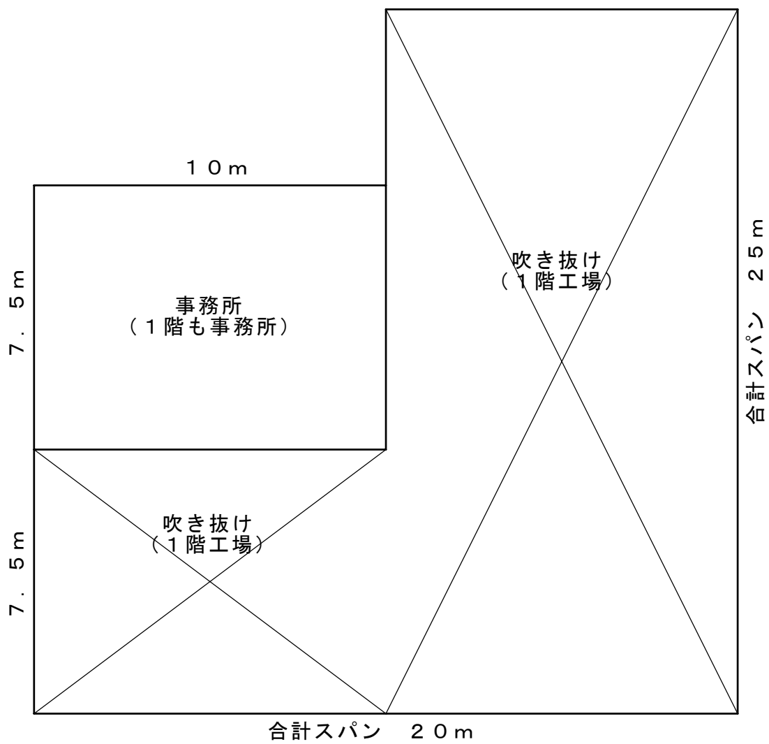
2階平面図
