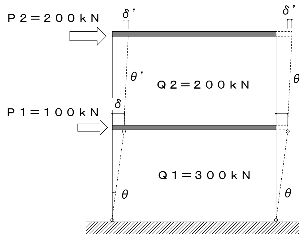
⑤のときの限界荷重状態
