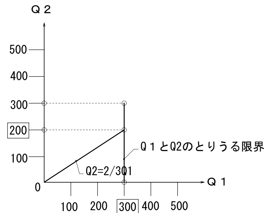
④、⑤ Q_1 : Q_2 = 2 : 3 のとき
