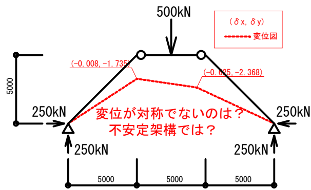
モデル②(ピン)
