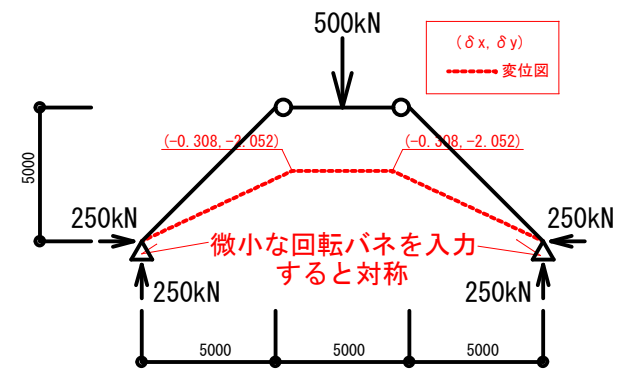
モデル③(ほぼピン)
