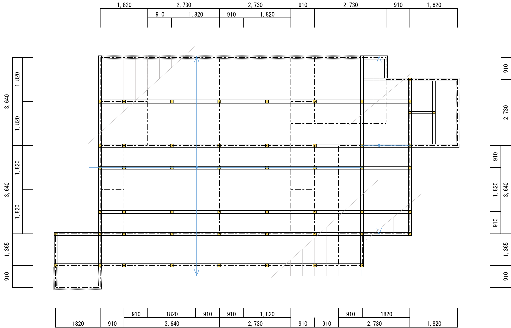
屋根伏図
